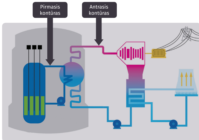
„Rosatom“ VVER tipo reaktorių modelis rosatomnewsletter.com
